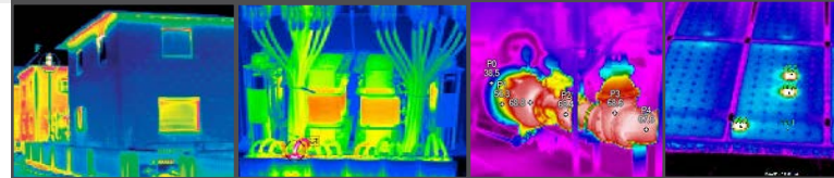
popis obr. zleva: tepelné mosty, elektrický rozvaděč, rozvody tepla v kotelně, vadné fotovoltaické panely
